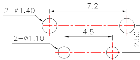
PCB Layout(Pattern side)
