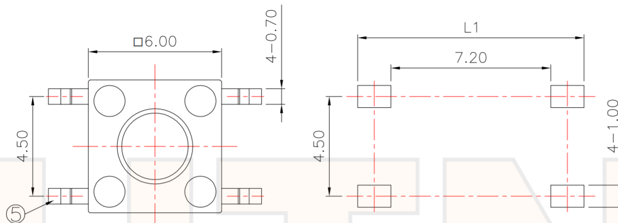
PCB Layout(Pattern side)
