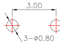
PCB Layout(Pattern Side)
