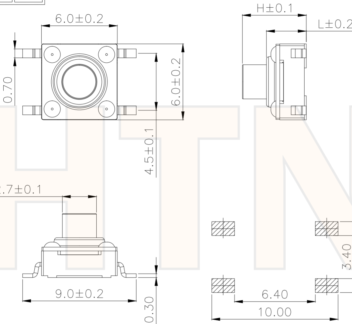
PCB Layout(Pattern side)
